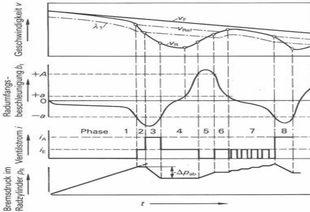
Instabilitätsregler (-logik) mit Beschleunigungsschwellen
