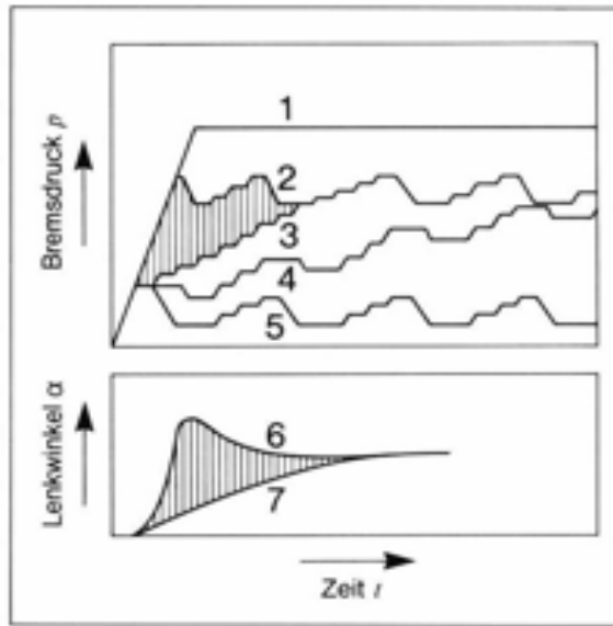
GMA: Bremsdruck-/Lenkwinkelverlauf 1 Hauptbremszylinderdruck p_{HZ} , 2 Bremsdruck p_{high} ohne GMA, 3 p_{high} mit GMA 1, 4 p_{high} mit GMA 2, 5 p_{low} , 6 Lenkwinkel \alpha ohne GMA, 7 Lenkwinkel \alpha mit GMA.
