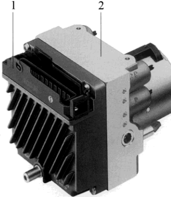
1: Hydroaggregat mit Anbausteuergerät
